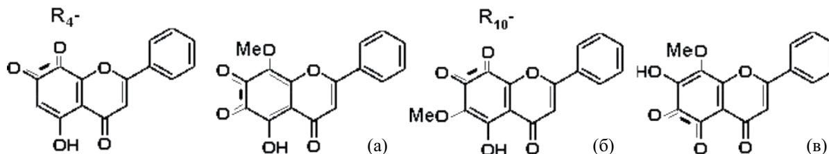
Рис. 5. Схемы редуктантов R_4^- m/z 268 и R_{10}^- m/z 298 при активации столкновением ионов [M-H]^- флавонов 4 и 10 в источнике ионов. (а, б, в) —предполагаемые структуры 6-ОМе вогонина.
