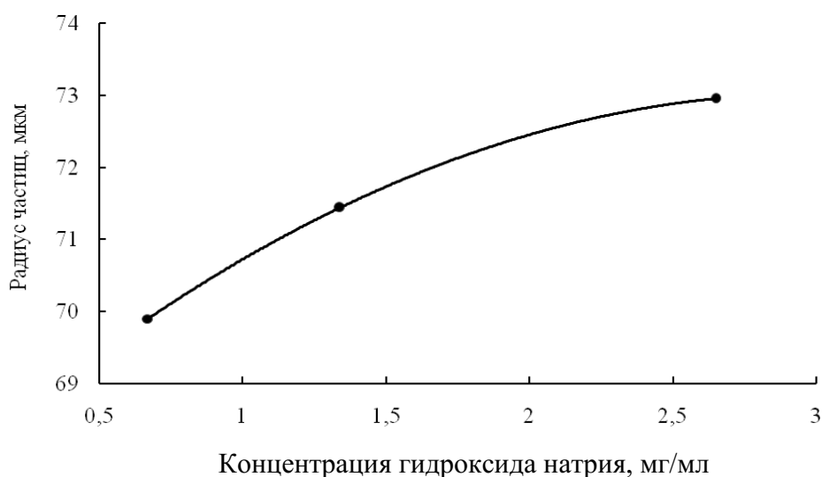
Рис. 1. Зависимость радиуса частиц осадка от содержания гидроксида натрия в сточных водах с концентрацией ионов никеля 1,174 мг/мл
