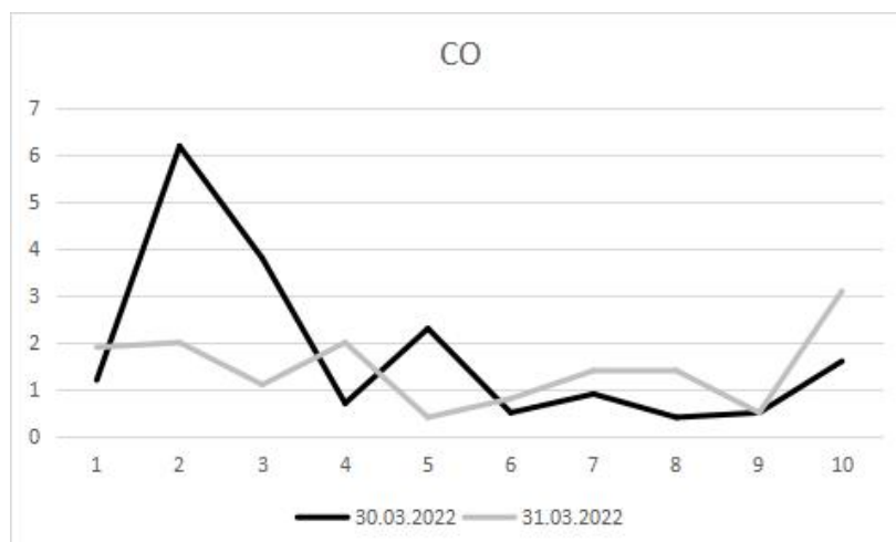
Рис. 2. Содержание угарного газа в воздухе, мг/м 3
