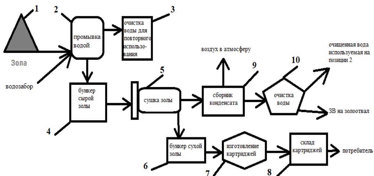
Рис. 3. Технологическая схема производства картриджей.
