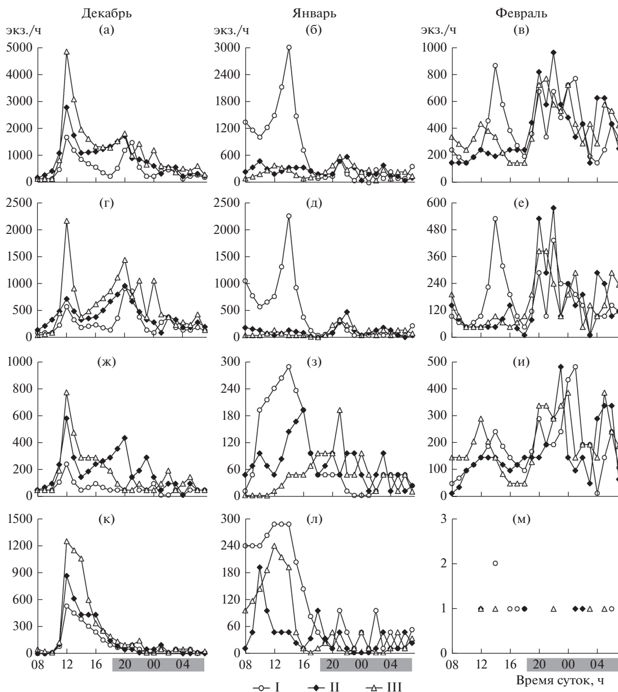
Рис. 2. Интенсивность дрейфа донных беспозвоночных на разных горизонтах в течение суток: все группы (а–в), Ephemeroptera (г–е), Diptera (ж–и), Hydracarina (к–м). I, II и III – придонный, срединный и поверхностный горизонты. Темная заливка – темное время суток. На рис. (м) показаны первичные данные.
