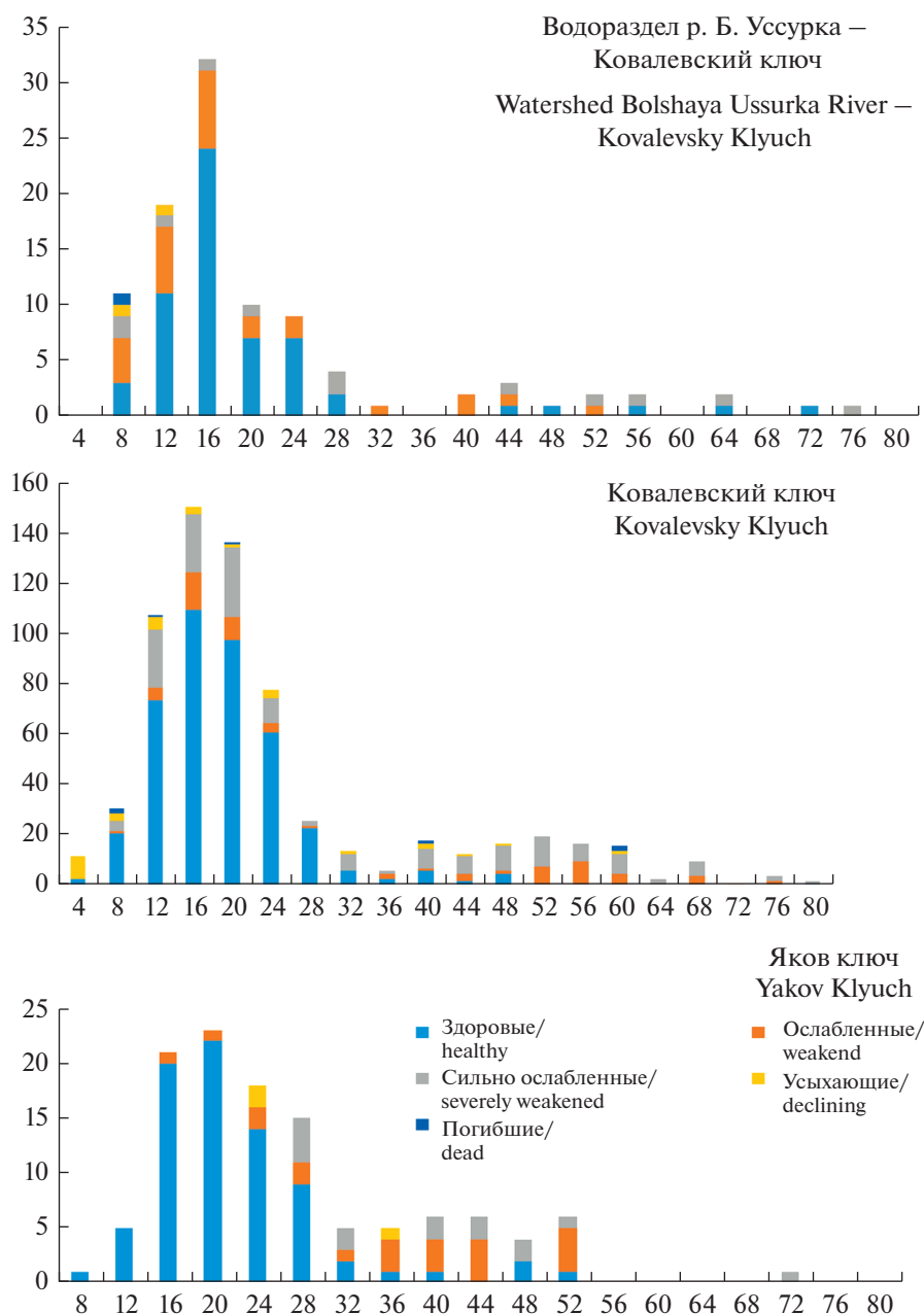
Рис. 2. Распределение Taxus cuspidata по категориям санитарного состояния в зависимости от диаметра. Данные по ключам Николаев и Трофимов не приводятся из-за малочисленности тиса.
